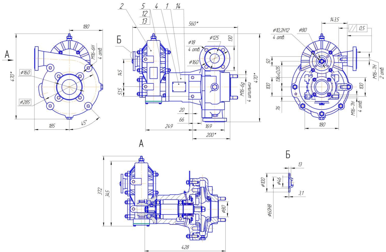
Рис. 1 Насос центробежный НЦ-60/125АП-01Р
