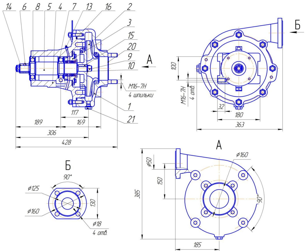
Рис. 2 Насос центробежный НЦ-60/125АП-01Б
