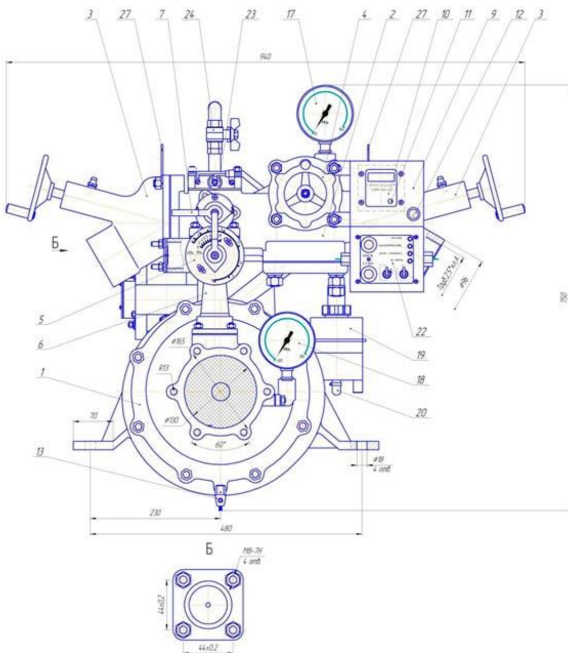
Рис. 1 Насос пожарный НЦПН-40/100УВМ.Э24
