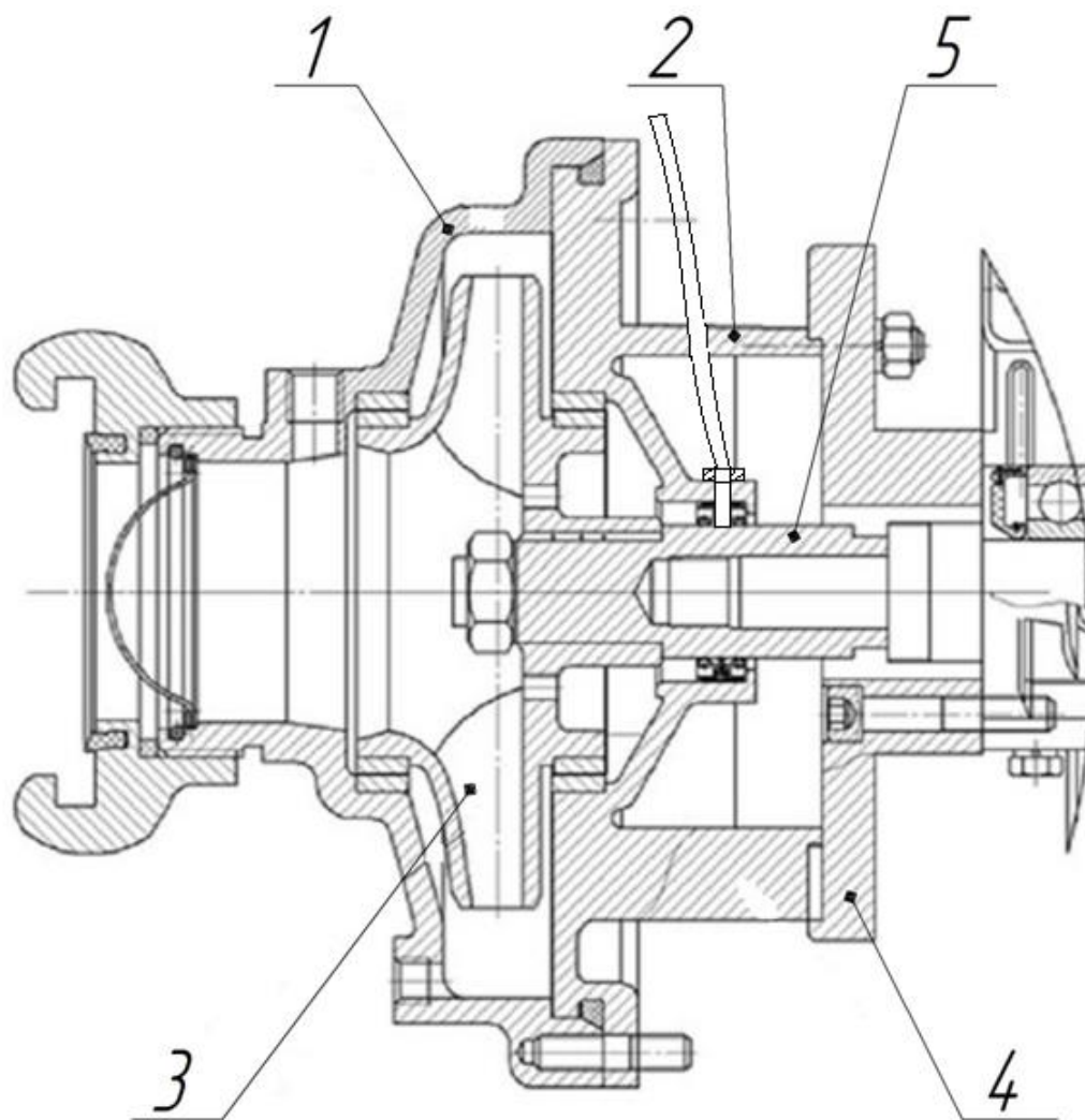
Рис.3 – Насос центробежный.
