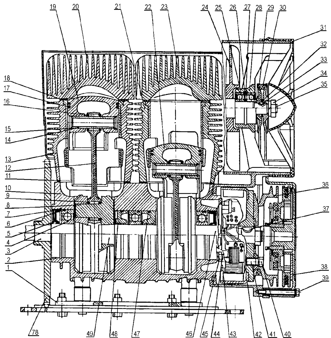
Рис. 1 – Двигатель
