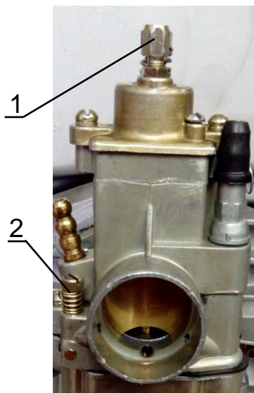
Рис. 19 – Регулировка карбюратора К65В
