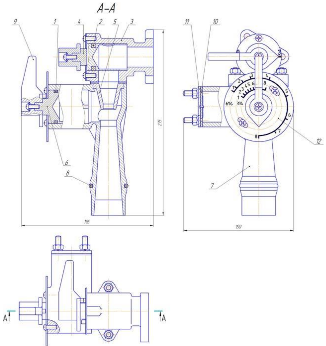
Рис.4 Пеносмеситель ПС-8
