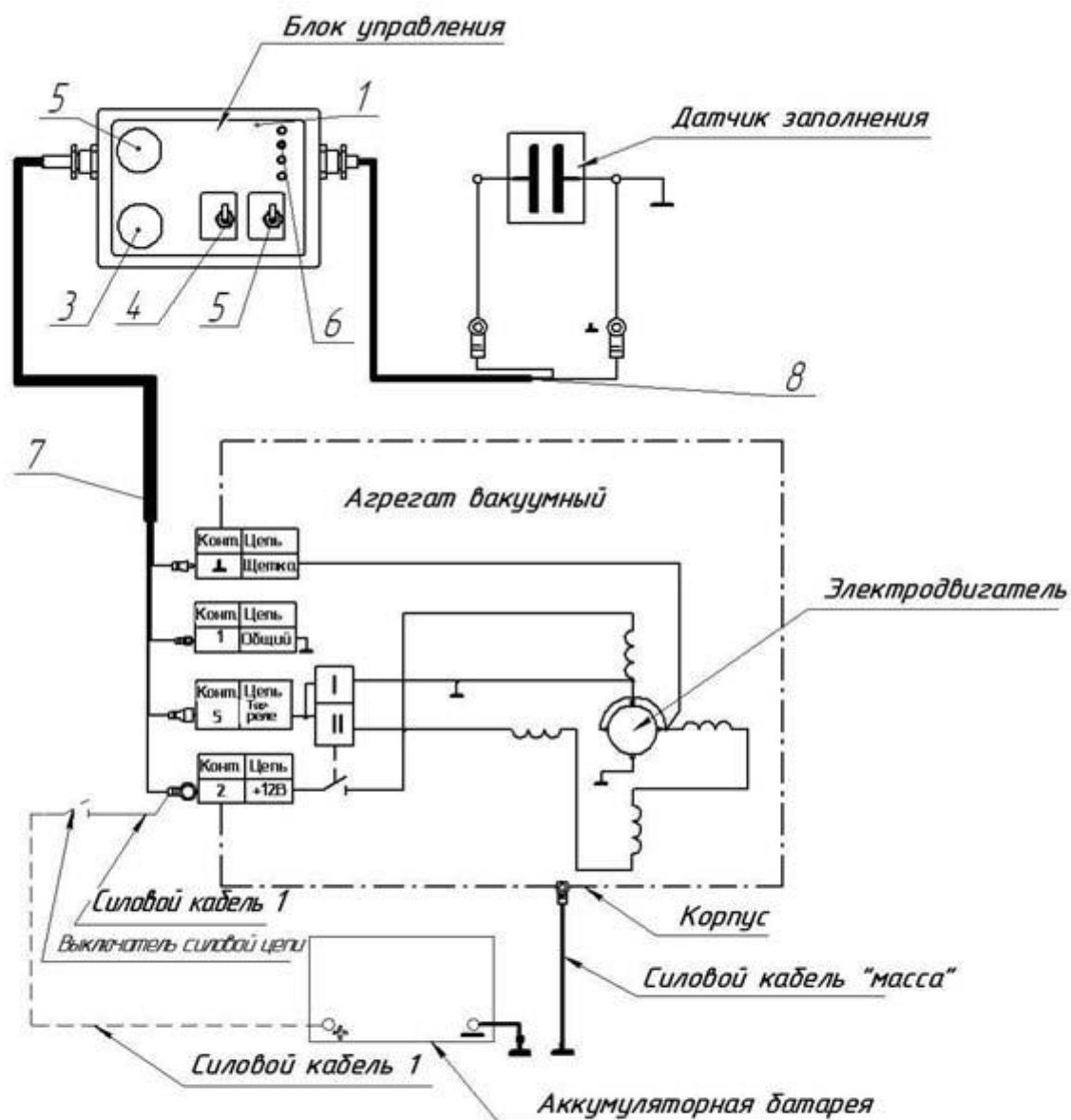
Рис. 5 Схема электрическая
