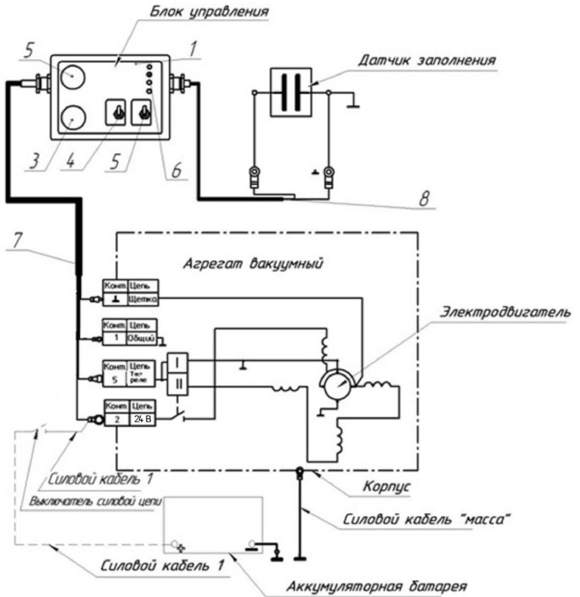
Рис.5 Схема подключения блока управления
