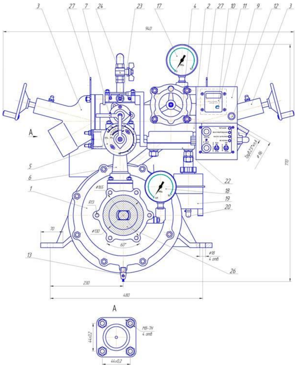
Рис. 1 Насос пожарный ПН-40УВ.324
