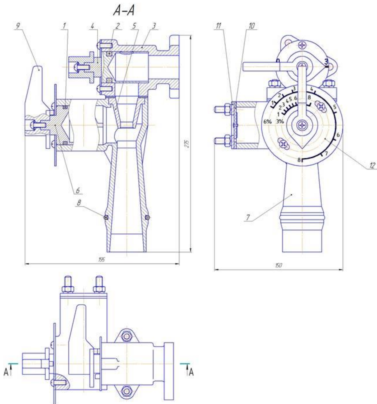
Рис.4 Пеносмеситель ПС-8
