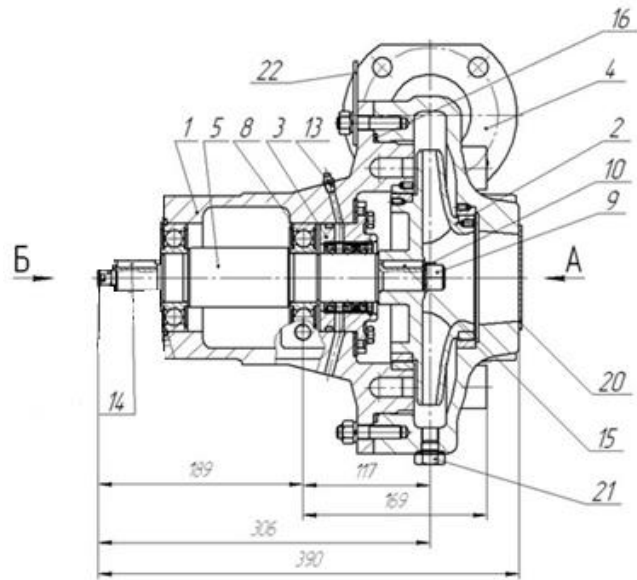
1-корпус насоса, 2-колесо рабочее, 3-стакан, 4-кронштейн, 5-вал, 8-подшипник, 9-гайка, 10-шайба, 13-масленка, 14-шпонка, 15-шпонка, 16-кольцо, 20-заглушка, 21-пробка, 22-кронштейн.
